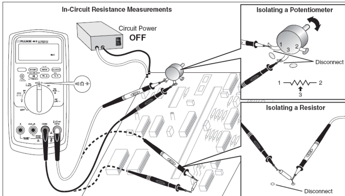
图 4.测量电阻
