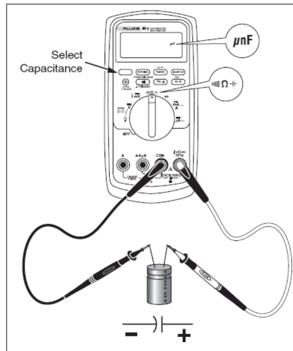
图 5.测量电容
