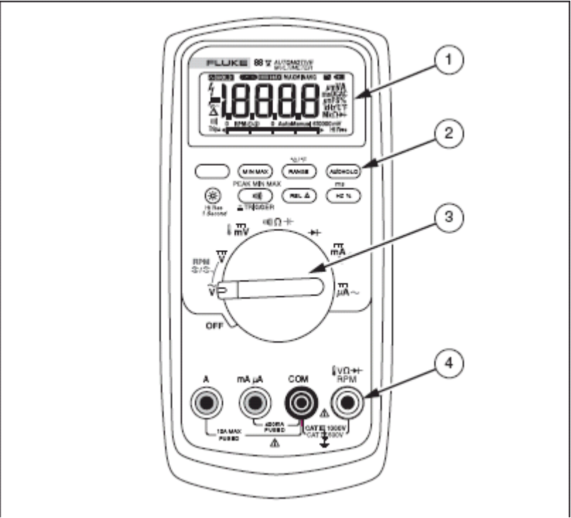
图-1 88V 型万用表前侧面板
