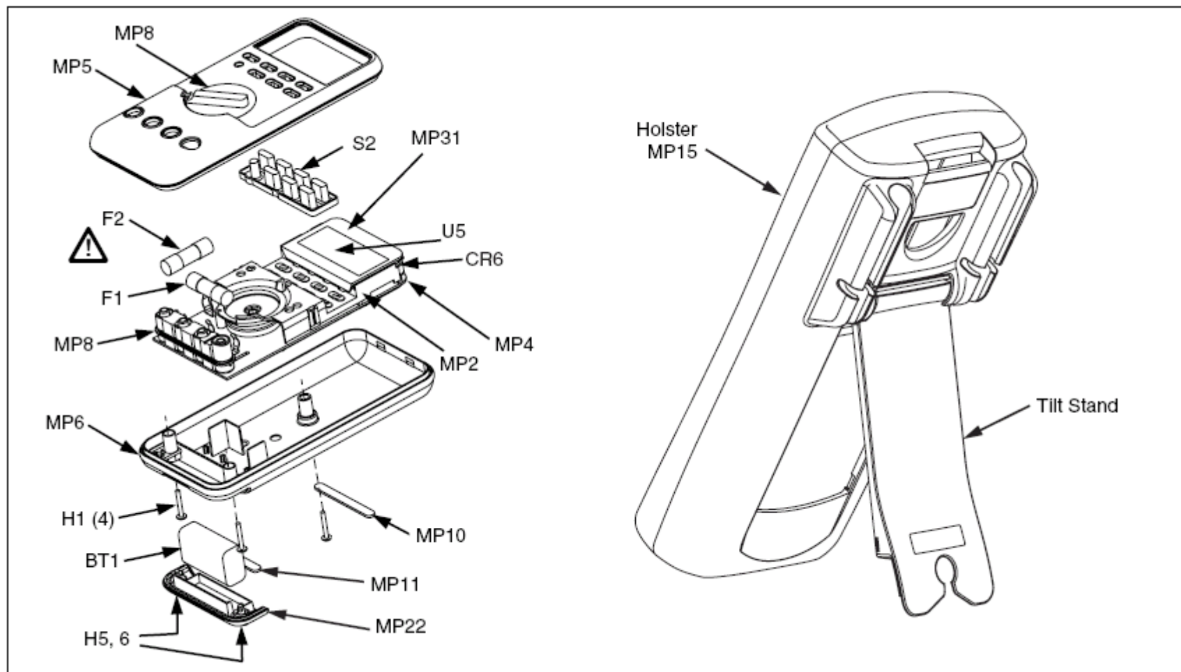
图 22.可更换零件
