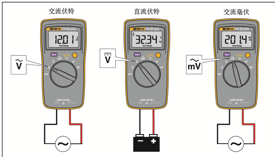
图 3. 测量交流电压和直流电压
