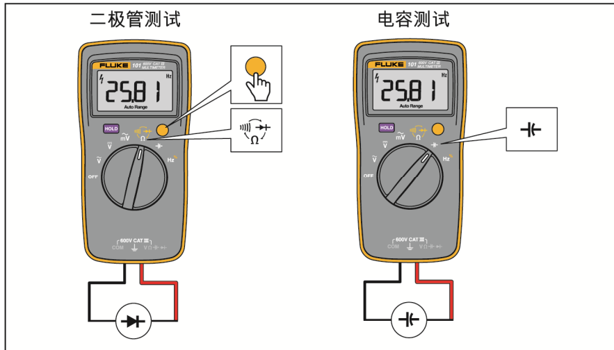
图 5. 二极管和电容测试
