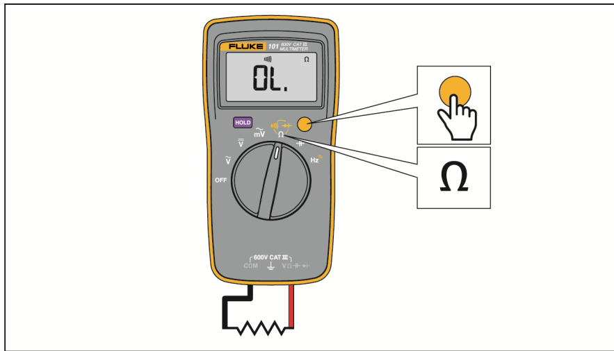
图 4. 测量电阻/通断性
